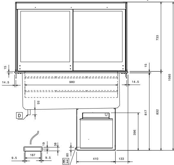
Zij aanzicht
